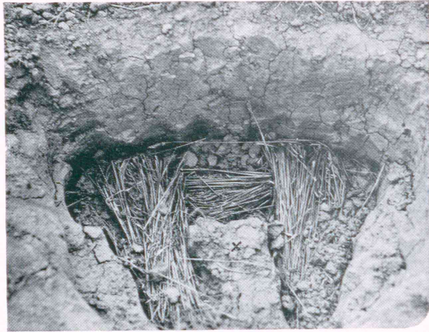
各個膝射散兵壕 (す下を腰に部出突の印×みつを膝兩)
